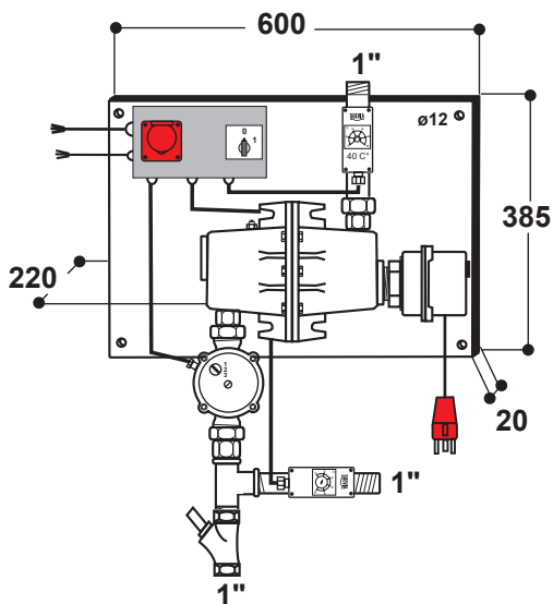
Abmaße • Dimensions • Габариты Mod. 311
