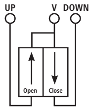
Tilkoblingsklemmer for eksterne taster
